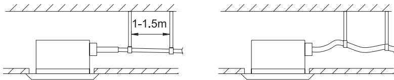
√ (Correcto) Inclinación de 1/100 o más
